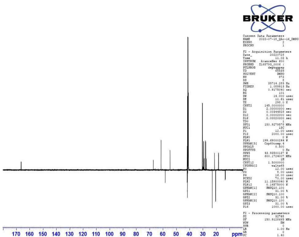
Slika 55. ^{13}\text{C} NMR spektar QAc- \text{C}_{16} .
