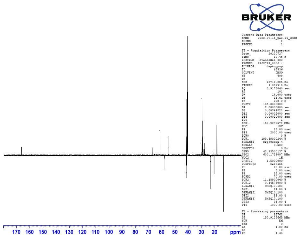
Slika 53. ^{13}\text{C} NMR spektar QAc- \text{C}_{14} .
