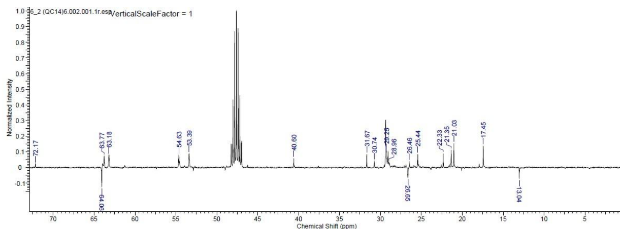
Slika 85. 13 C NMR 2(QC 14 ) 6 .
