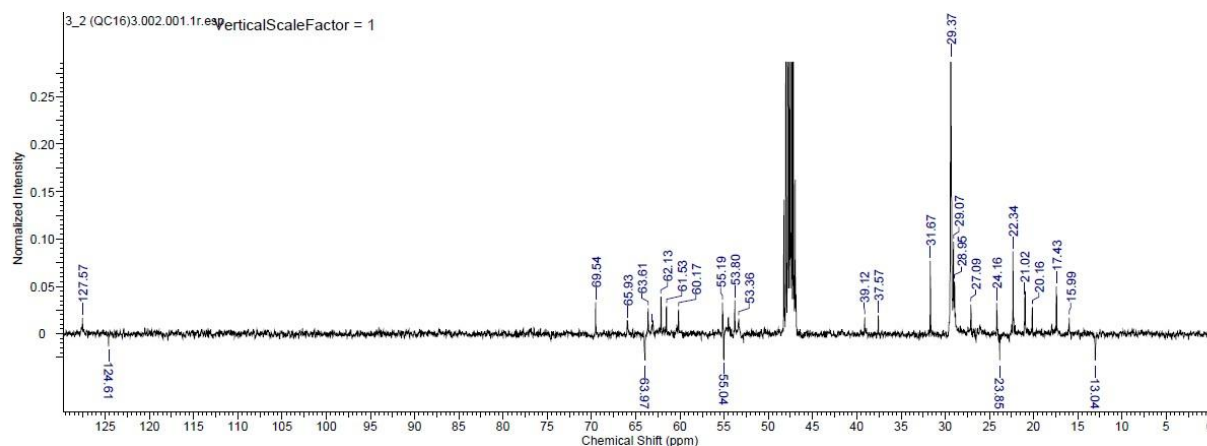
Slika 75. 13 C NMR 2(QC 16 ) 3 .
