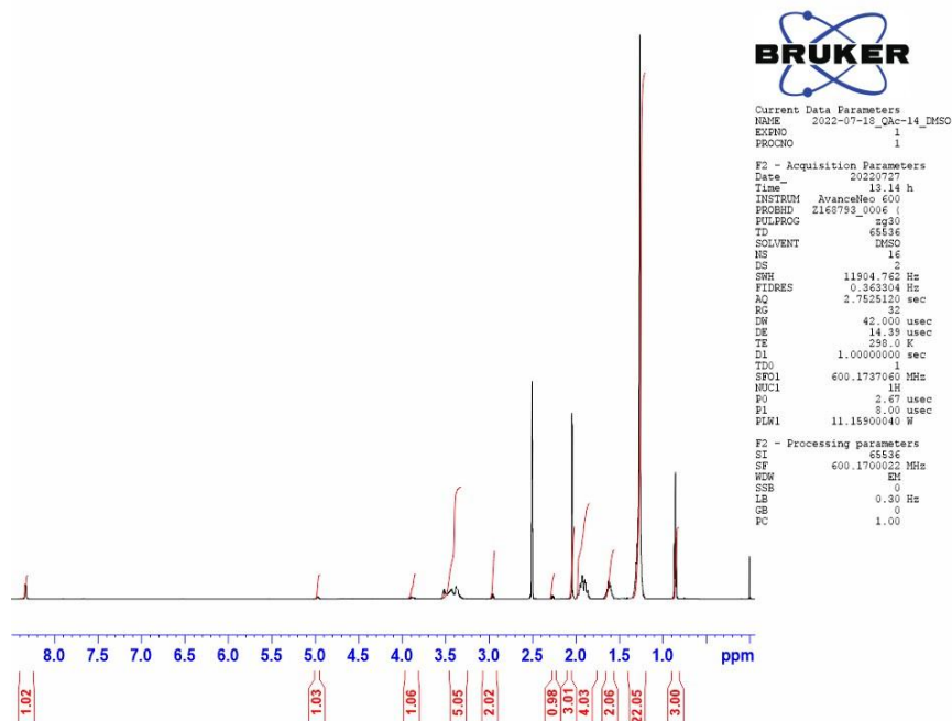
Slika 52. ^1\text{H} NMR spektar QAc- \text{C}_{14} .
