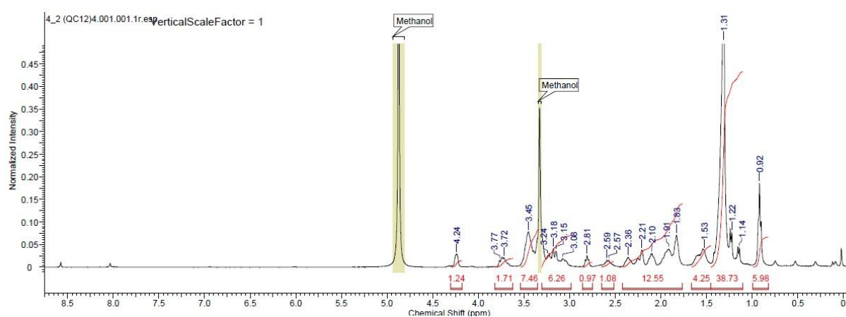
Slika 76. 1 H NMR 2(QC 12 ) 4 .
