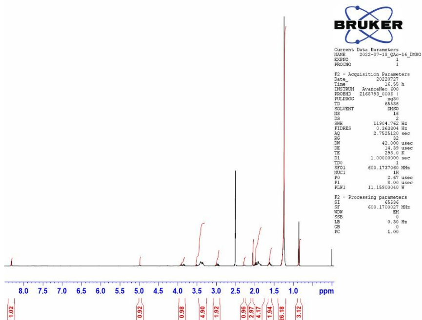
Slika 54. ^1\text{H} NMR spektar QAc- \text{C}_{16} .
