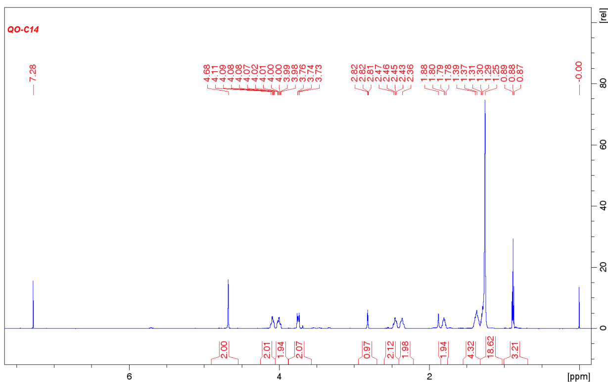
Slika 63. ^1\text{H} NMR spektar QO-C 14 .
