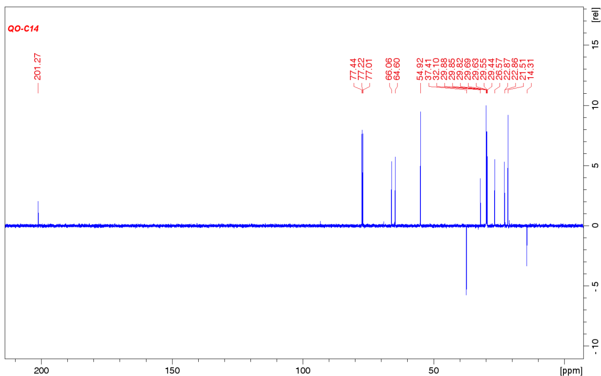
Slika 64. ^{13}\text{C} NMR spektar QO-C 14 .
