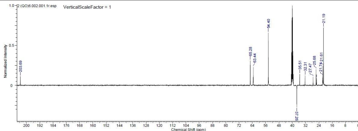
Slika 69. ^{13}\text{C} NMR 2(QO) 6 .
